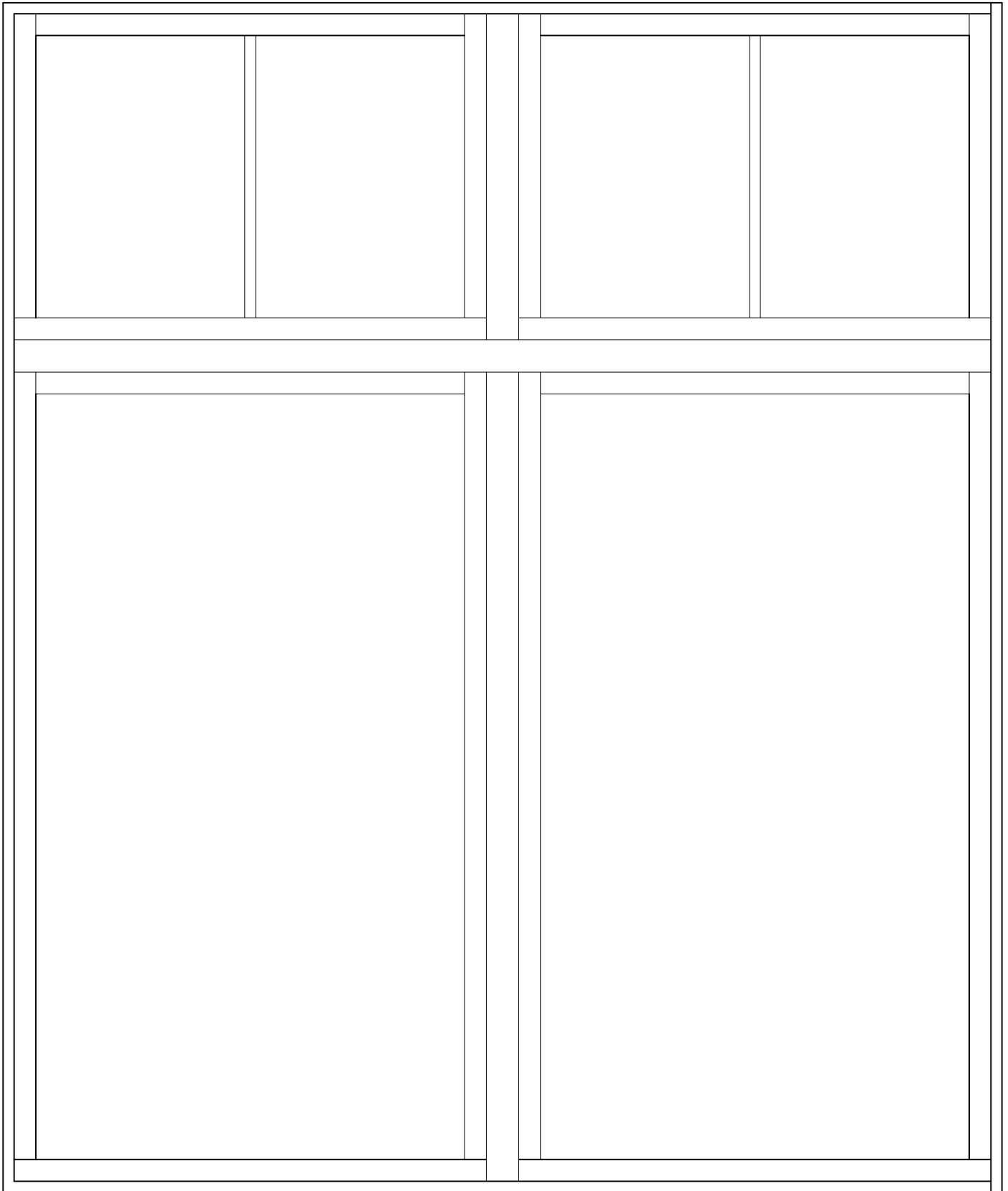
Widok nowo projektowanego okna D od frontu, skala 1:10
